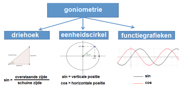
FIGUUR 10. Verschillende representaties bij goniometrie.
