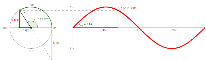
FIGUUR 2. Schermafdruck van GeoGebra activiteit voor sinusberekening via de eenheidscirkel-methode. Door het punt P te verslepen kan de draaiingshoek \alpha ingesteld worden en het bijpassende punt S op de sinusgrafiek gevisualiseerd worden.
