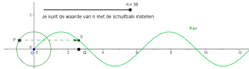
FIGUUR 9. Grafiek van de sinusachtige functie s_{30} bij een regelmatige 30-hoek.
