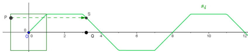
FIGUUR 6. Schermafdruck van een GeoGebra activiteit waarin de grafiek van een sinusachtige functie getekend is en de connectie tussen het punt P op de regelmatige vierhoek en het punt S op de grafiek van de verticale positie van P uitgezet tegen afgelegde afstand van het punt P gevisualiseerd wordt. Het punt Q op de horizontale as correspondeert met de afgelegde weg. De grafiek hoort bij een functie aangeduid met s_4 .
