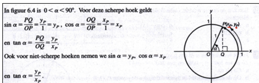
FIGUUR 3. Fragment uit een wiskundeboek waarin de overgang van driehoek naar eenheidscirkel toegelicht wordt.
