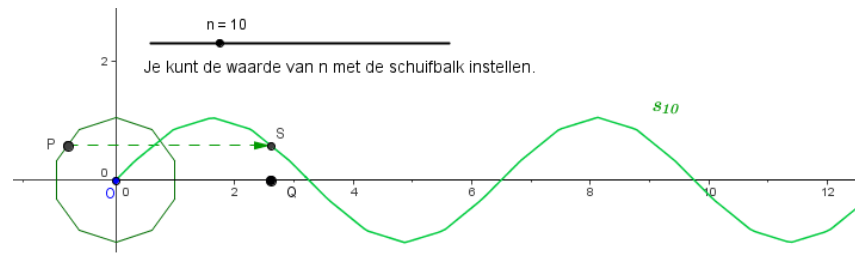
FIGUUR 8. Grafiek van de sinusachtige functie s_{10} bij een regelmatige 10-hoek.
