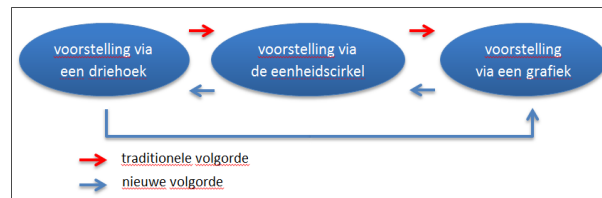
FIGUUR 11. Traditionele versus alternatieve aanpak van goniometrie.
