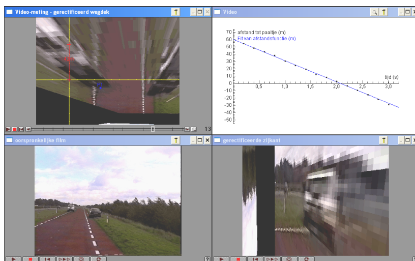
fig 8. Snelheidsbepaling van een auto m.b.v een gerectificeerde videoclip
