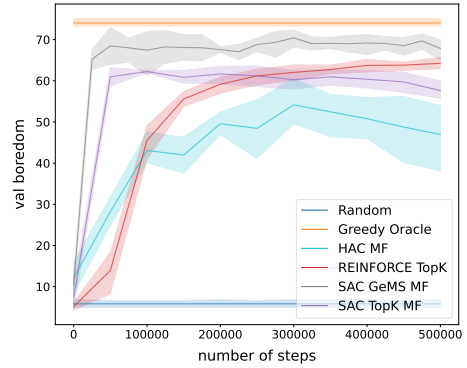
(d) Boredom (↓) on SlateTopK-Bored (MF)
