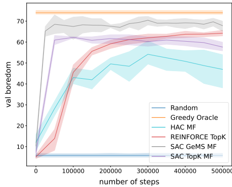
(d) Boredom ( \downarrow ) on SlateTopK-Bored (MF)
