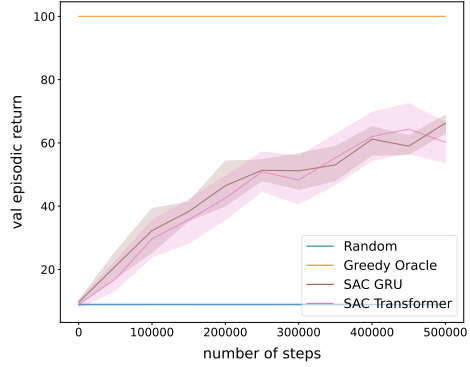
(b) Return (↑) on SingleItem-PartialObs
