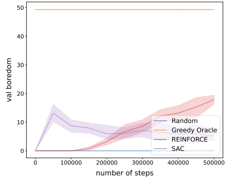
(d) Boredom (↓) on SingleItem-BoredInf
